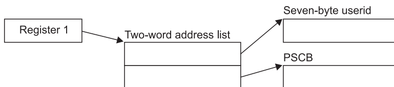
Figure 24. ERBT SOCK Input Parameter Structure
