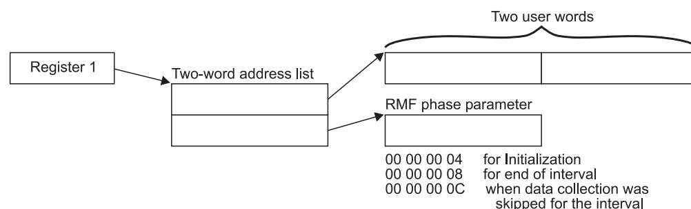
Figure 13. ERBMFDUC Input Parameter Structure
