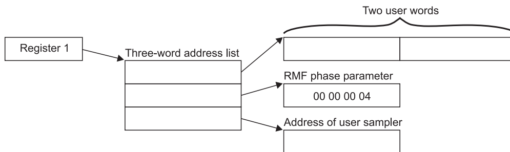
Figure 11. ERBMFIUC Input Parameter Structure
