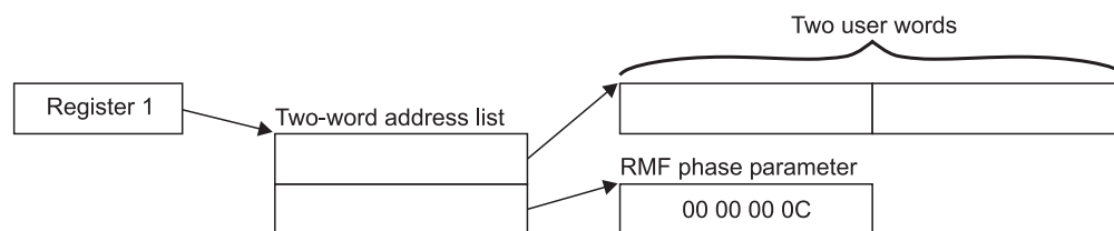
Figure 15. ERBMFTUR Input Parameter Structure
