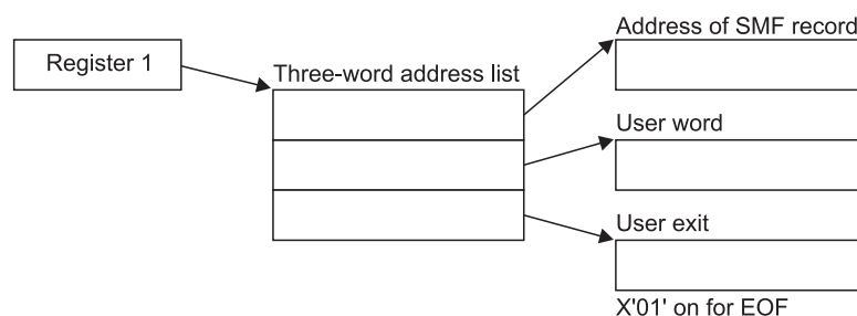
Figure 18. ERBMFPUS Input Parameter Structure
