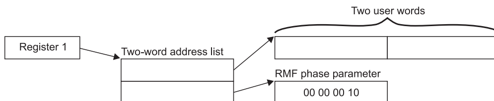
Figure 14. ERBMFRUR Input Parameter Structure
