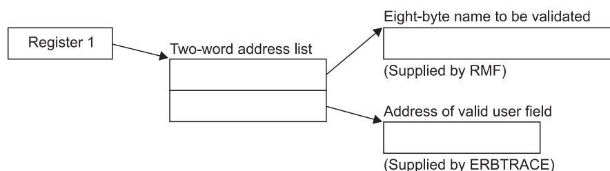
Figure 17. ERBTRACE Input Parameter Structure
